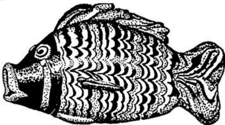
Рис. 42. Бутылка в форме нильской рыбы из белого, желтого, черного и синего стекла. Амарна, теперь хранится в Британском музее. Приблизительно 1350 г. до н. э. Длина 3 1/4 дюйма
